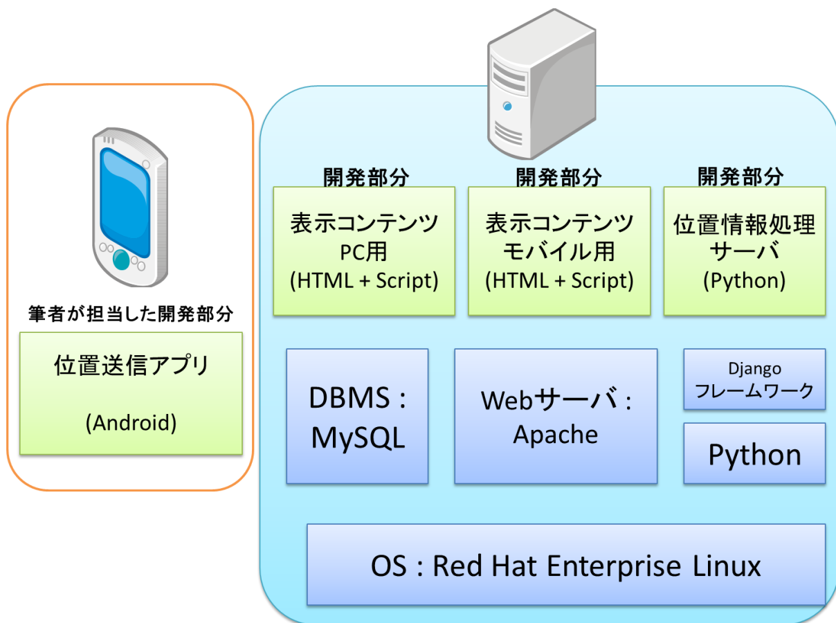
図 6 ソフトウェア構成
