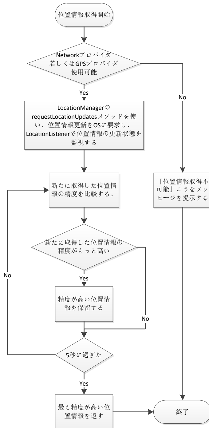
図 16 筆者が作ったアプリの位置情報取得のフローチャート
