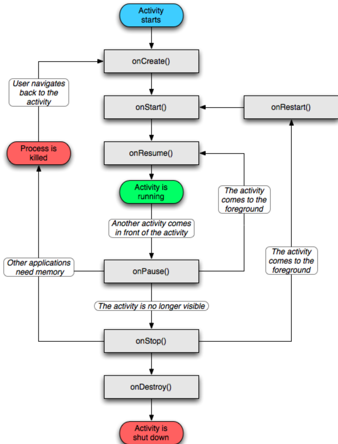
図 9 Activity のライフサイクル(Android API から引用)
