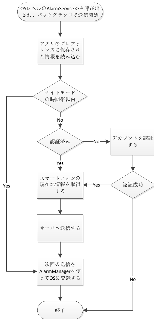
図 15 定期的にバックグラウンド送信のフローチャート
