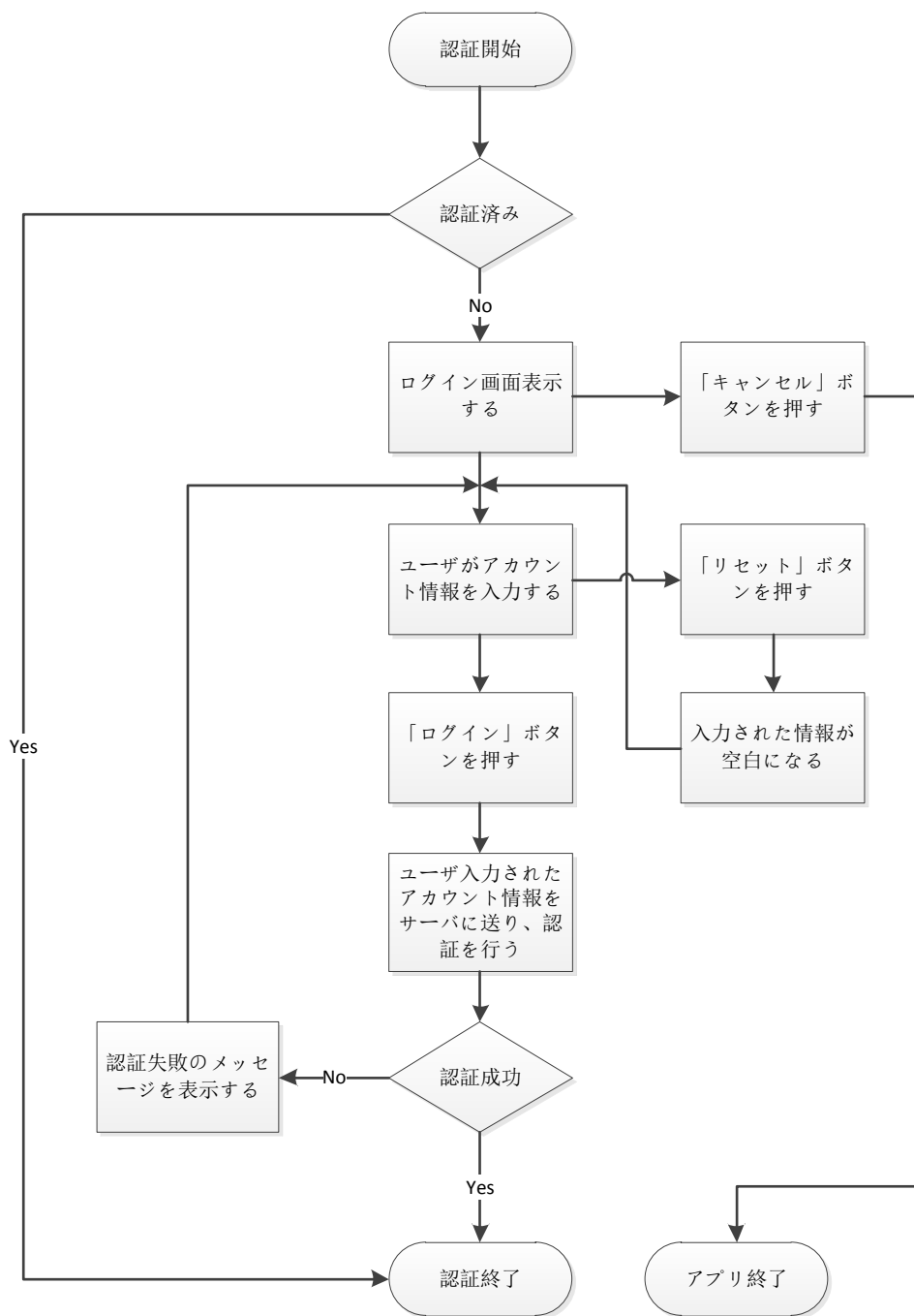
図 12 アカウント認証のフローチャート
