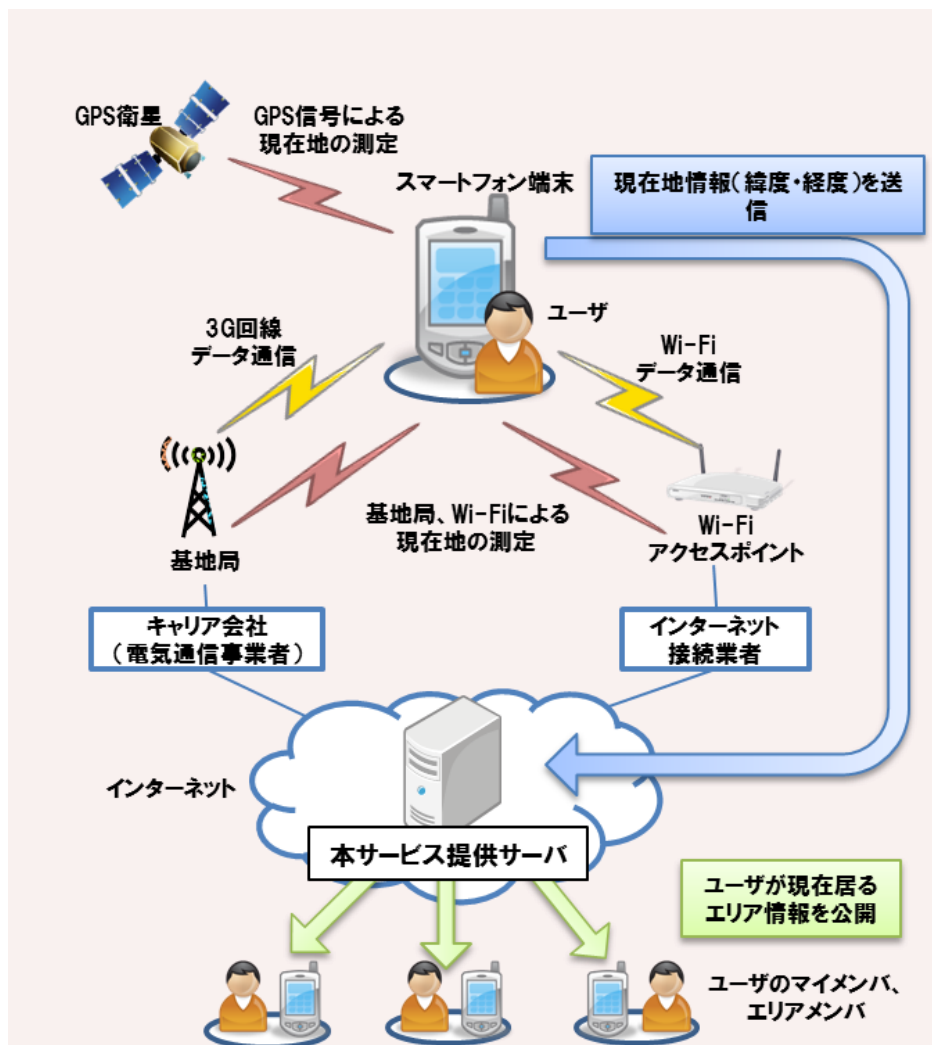
図 5 ハードウェア・ネットワーク構成
