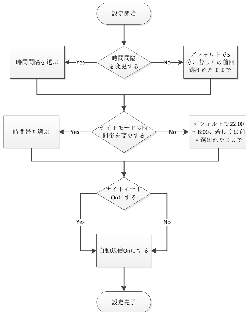
図 14 筆者が作った Android アプリ設定のフローチャート
