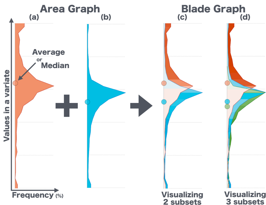
図 4.1: Blade Graph の生成例。
