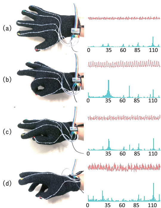
図 5. 指同士が接触した際の応答波形 (赤線) および周波数スペクトル (青線)
