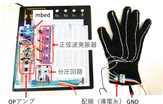
図 4. 手形状計測用回路
