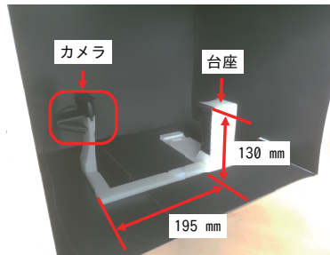
図 7. 実験に用いた台座および箱
