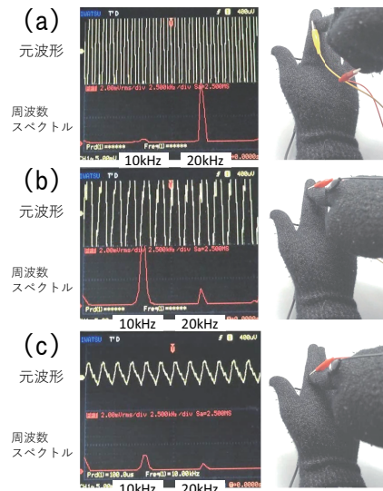
図 10. 両手の指が接触した際の応答波形（右手の人差し指に10kHz、中指に20kHzの信号を印加）
