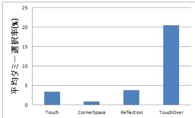
図 18 実験結果：ダミー選択率
