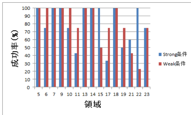
図 9 予備実験結果：識別成功率
