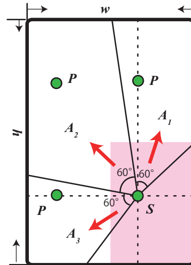
図 4 TouchOver におけるタッチ点及び転送後のタッチ点の位置の関係
