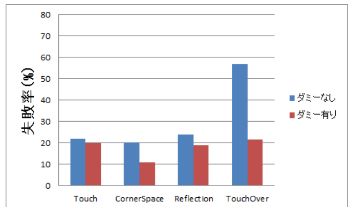
図 17 実験結果：理想起動状態での失敗率
