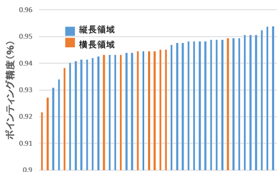
図 6 領域毎のポインティング精度（ソート済み） Fig. 6 Pointing accuracy on each area (sorted).
