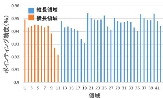
図 5 領域毎のポインティング精度 Fig. 5 Pointing accuracy on each area.
