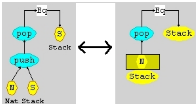
図 5.4: ビューの切替えと等式の表現
