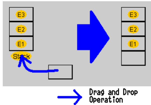
図 4.8: カスタマイズ後のビューを用いた項の編集（追加）
