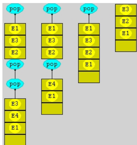
図 5.5: カスタマイズ表現を用いた実行表示
