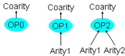
図 3.5: CafePie における演算の視覚化
