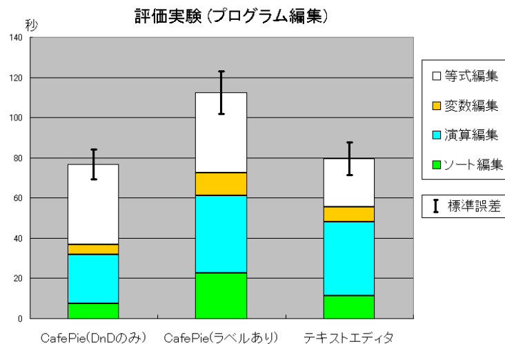
図 3.14: プログラム編集における評価
