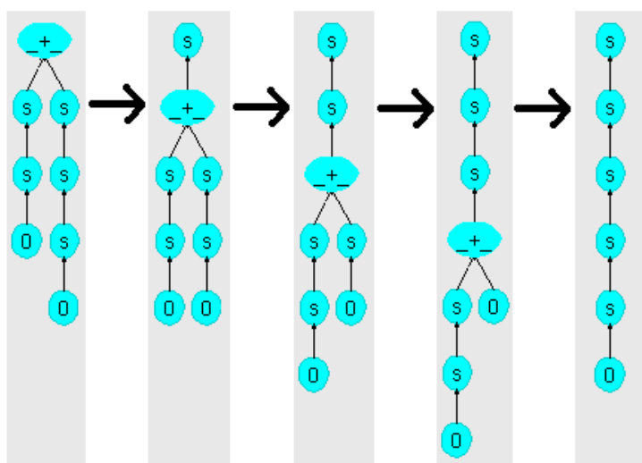
図 5.2: 動的な実行の視覚化
