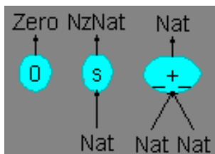
図 3.11: CafePie 上の演算定義例
