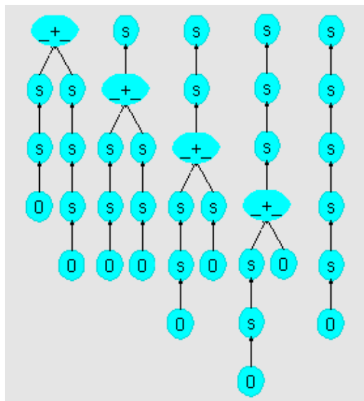
図 5.3: 静的な実行の視覚化
