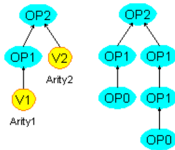
図 3.4: CafePie における項の表現
