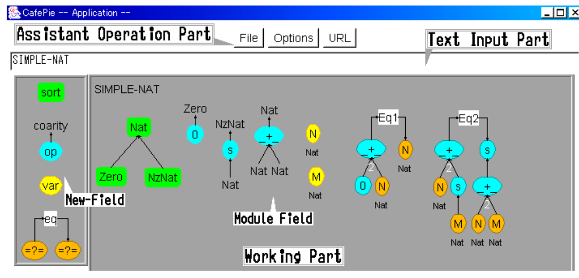
図 3.2: CafePie の実行画面
