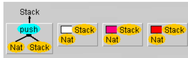
図5.16: 演算 push に定義したマルチビュー
