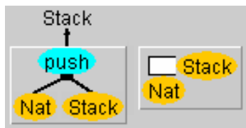
図 5.10: ソーティングでの演算 push 図 5.11: ソーティングでの演算 empty
