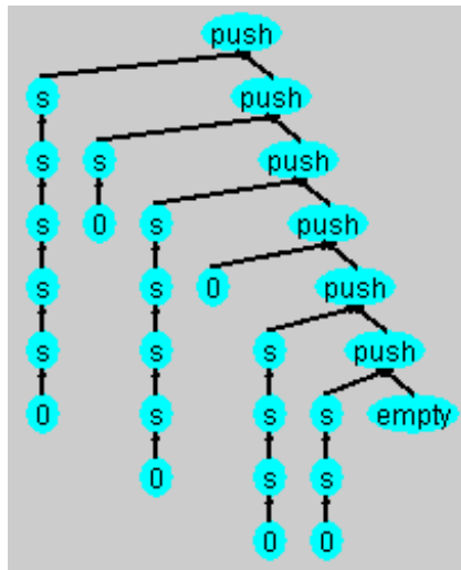
図 5.9: ソーティングにおけるゴール
