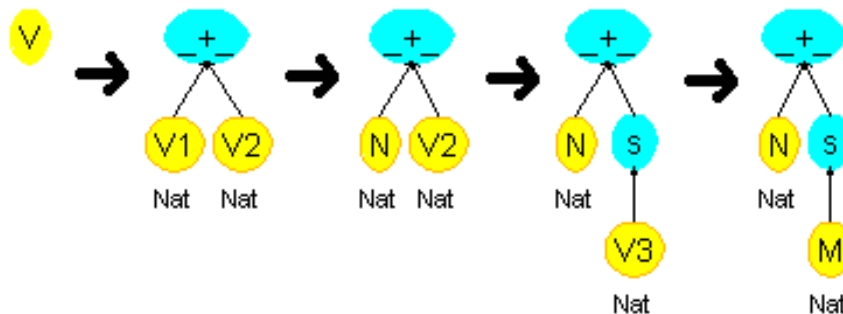
図 3.9: 項の作成手順
