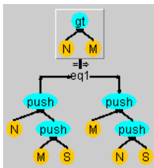
図 5.8: ソーティング用の等式
