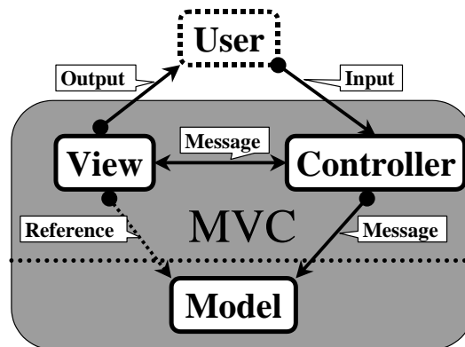
図 4.1: MVC モデル
