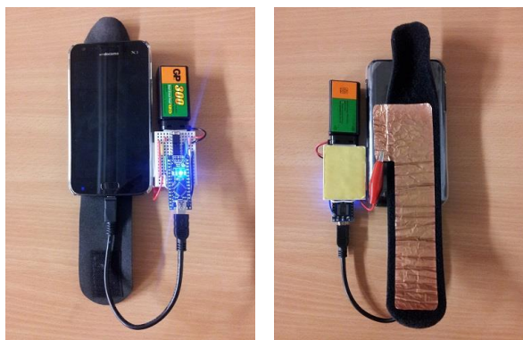
(a) 表側 (b) 裏側 図 2 : 試作したウェアラブルデバイス
